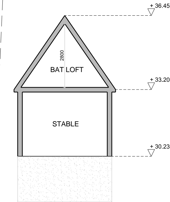
4. SECTION BB 1:100 @ A3
